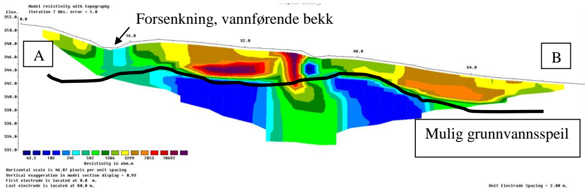
Figur 46 Profil av forsøksområde L.3. Vegetasjonsdekket består av fra (A) Barskog med overgang til Lauvskog (B). Svart linje deler høy resistivitet i overflaten til svært lav resistivitet under. Svart pil på venstre side (A) viser en forsenkning der det går en bekk.
