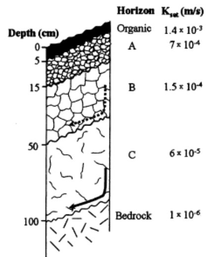
Figur 12 Typisk jordprofil med horisonter for skog i en skråning. Horisonter, ABCD og grunnfjell. Til høyre i figuren ( K ) vises hydraulisk konduktivitet. Lateral bevegelse er mest vanlig i C horisonten, og forekommer ved større nedbørshendelser i B horisonten. (Sidle & Ochiai, 2006).
