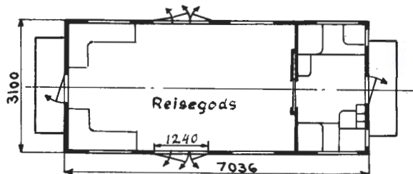
Grunnriss 1 Hovedt. B. 543
