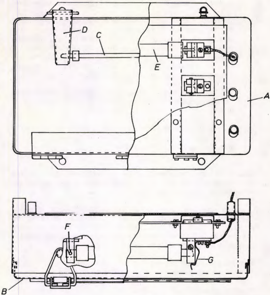
Fig. 4. 3-polet sikringskasse.
