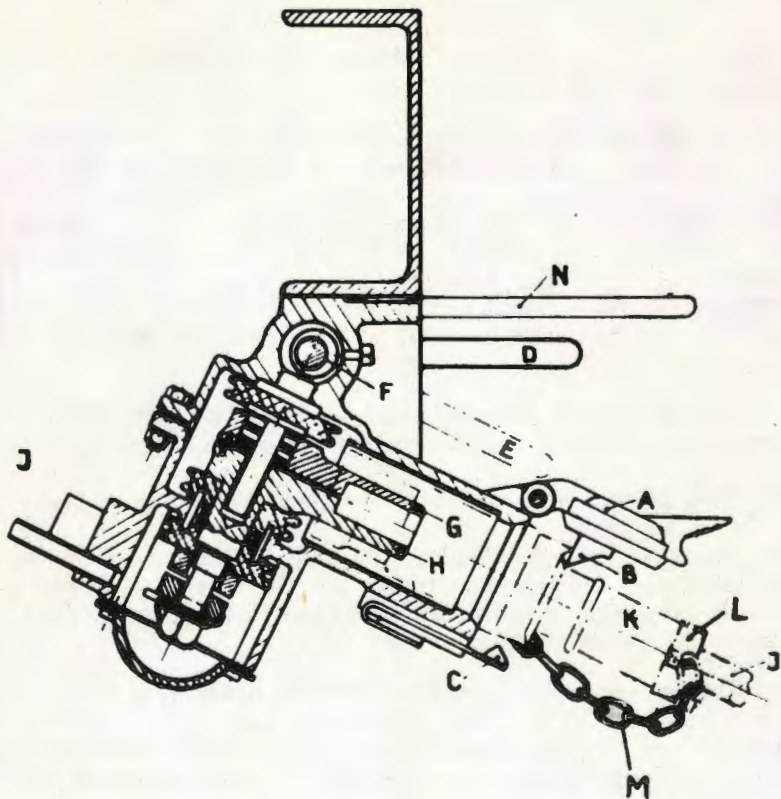
Fig. 5. Togvarmekontakt.
