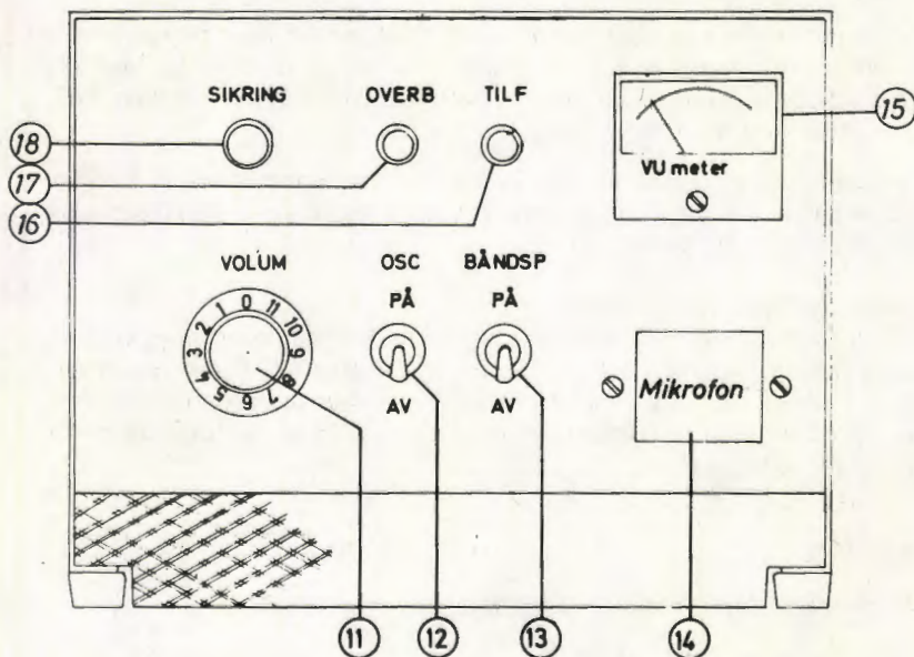
Fig. 1. Høyttalerforsterker «VINGTOR» type NA 3. Tallene viser til tekst i artikkel 3.1.
