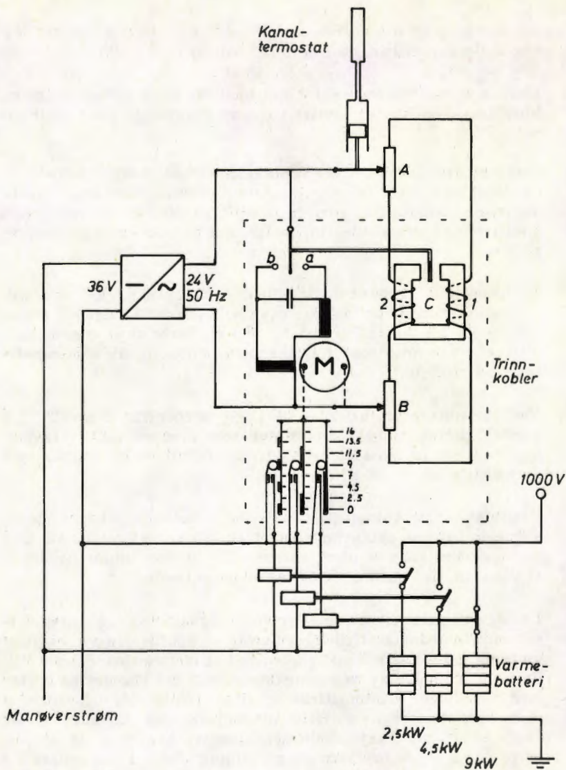
Fig. 10. Automatisk varmeregulering av ventilasjonsanlegg i personvagner litra WL og AB.
