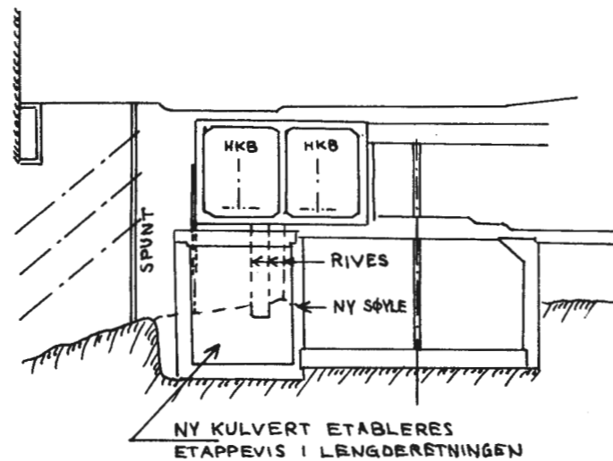
SNITT Km 1,085
