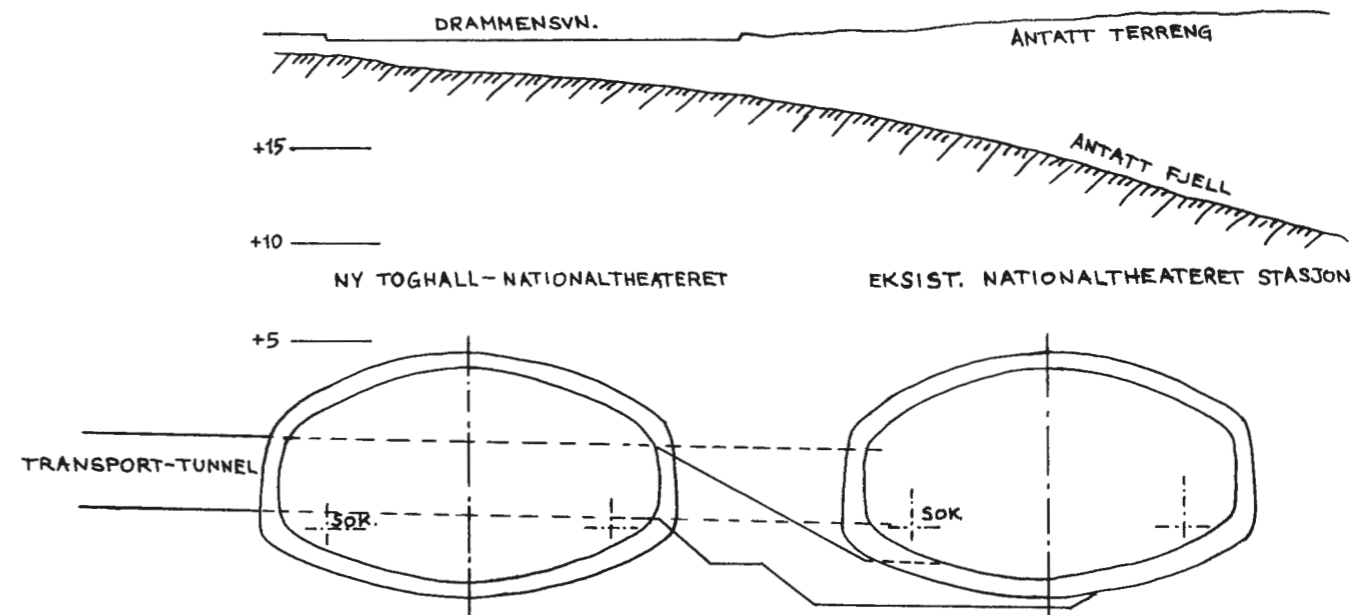
TYPISK SNITT VED STASJON
