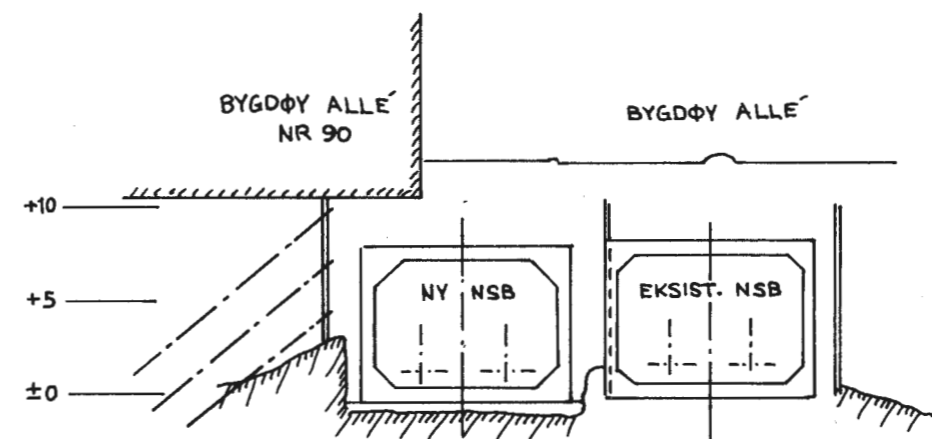
SNITT Km 3,415
