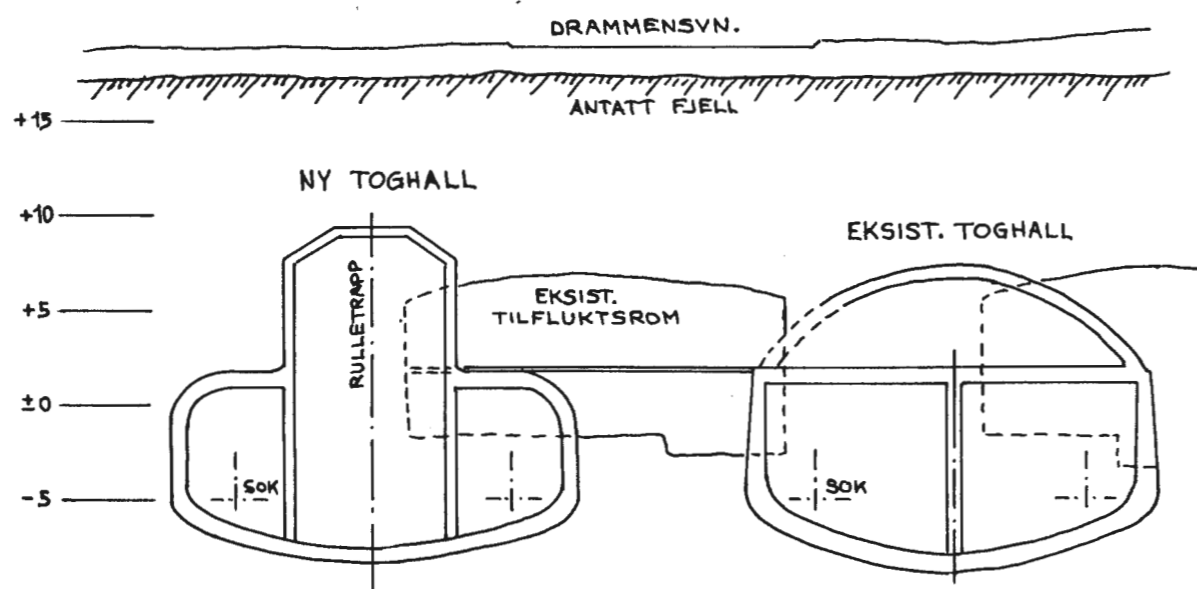
SNITT Km 1,305
