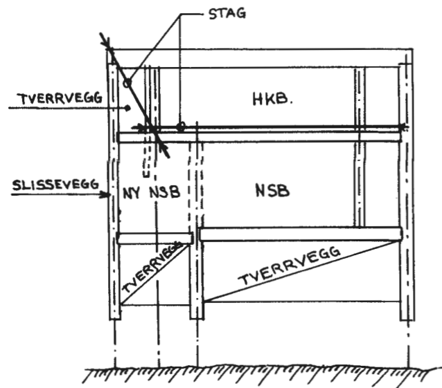
SNITT Km 1,060
