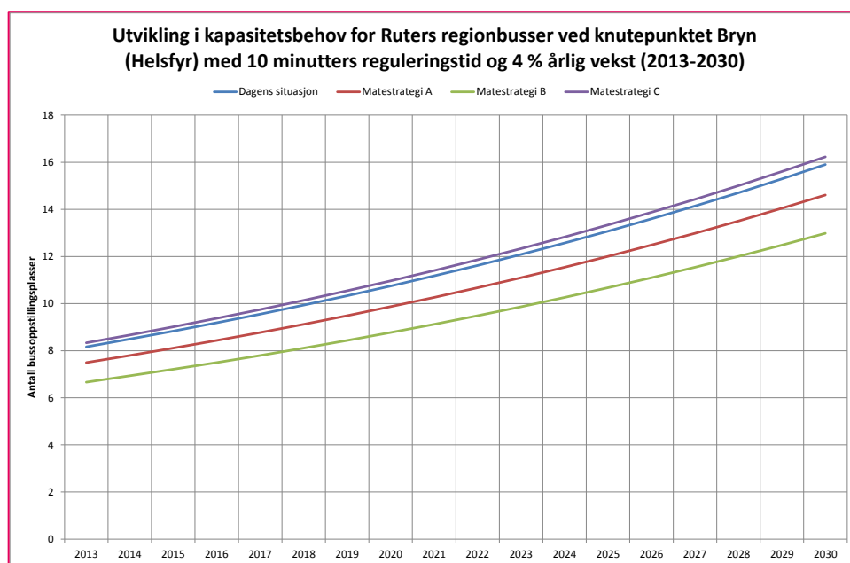
Figur 0.57: Estimert utvikling i kapasitetsbehov (antall bussoppstillingsplasser) for Ruters regionbusser ved knutepunktet Bryn (Helsfyr) ved 10 minutters reguleringstid (virkedag) ved alternative matestrategier og 4 prosent årlig vekst (2013–2030)
