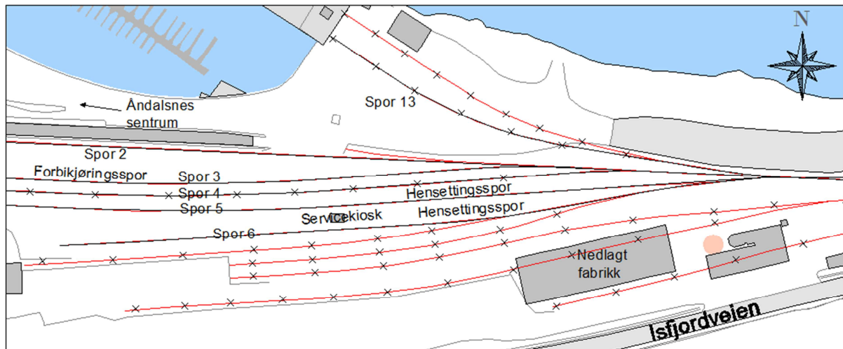
Figur 3: Viser spor som er i bruk i dag (svart), spor som er i dårlig stand men kan brukes (svart med kryss) og spor som ikke er i stand og ikke brukes (rødt med kryss)
