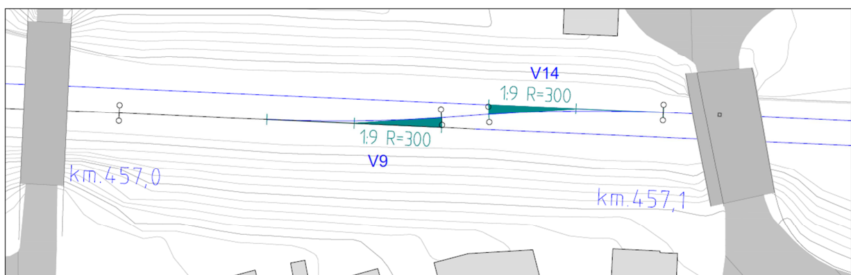
Figur 11: dobbeltspor, alternativ 1
