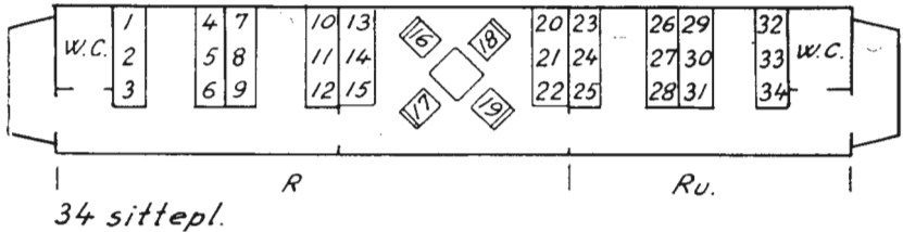
Bo 2c nr. 581
