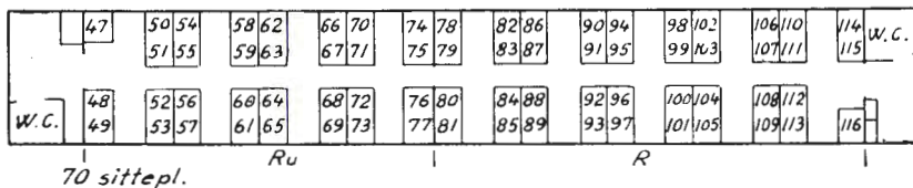
Bo 3e mellomvogn for BFmdo 88
