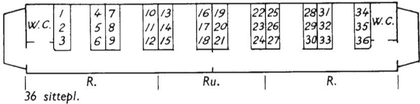
Bo 2c nr. 248, 811, 950.
