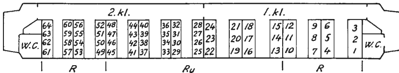
AB o 2 c (stål)
