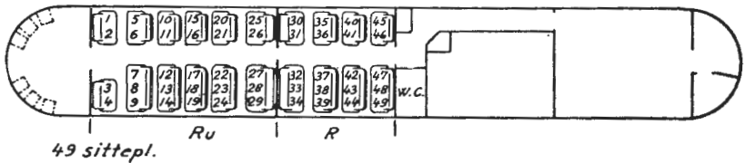
CDFox 4b Styrevogn for Cmdo type 6.
