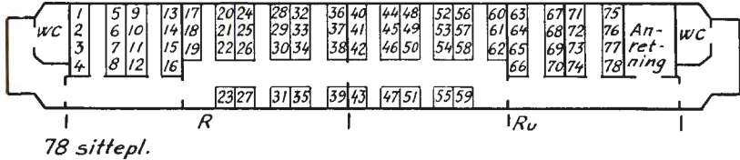
Bo 8ca (stål)
