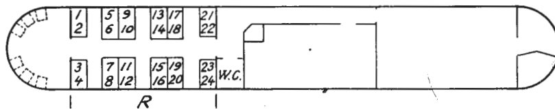
BDFox 3 - 11 styrevogn for Bmdo 86 og 91
