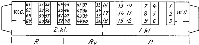
AB o 2 b
