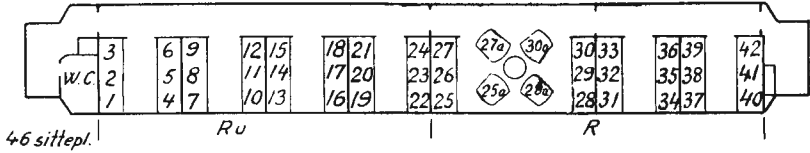
Ao 14c (stål)
