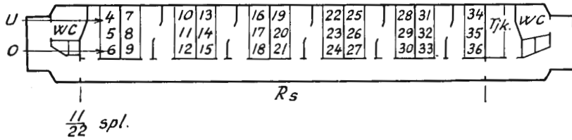
WLA o5a (stål)
