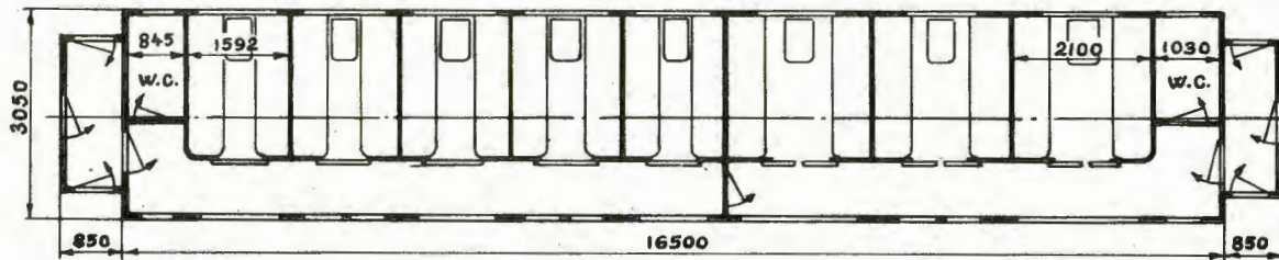
Hovedt, oppr. 699 + 869
