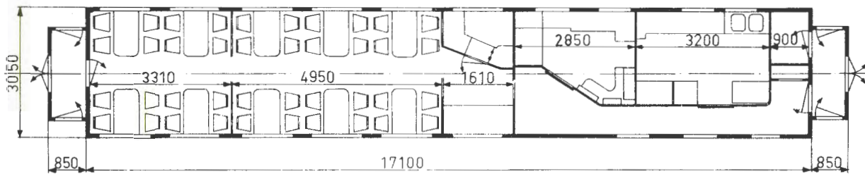
Hovedt. 2068 1)2)
