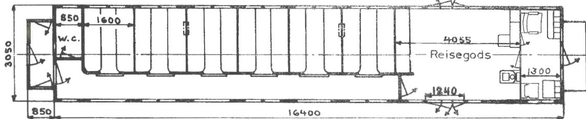
Mål i ( ) gjelder vogner etter grunnriss 2. og 3
