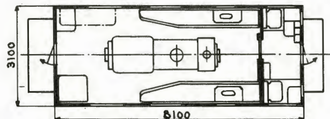
Grunnriss 2 Hovedt. 3043
