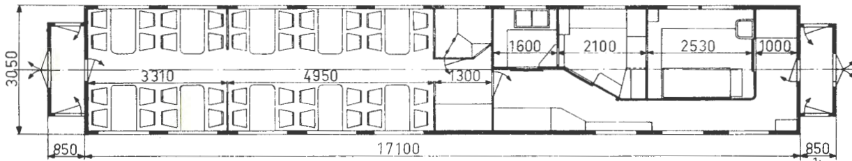
Hovedt. 1116 1)
