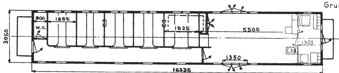
Hovedt. B.112
