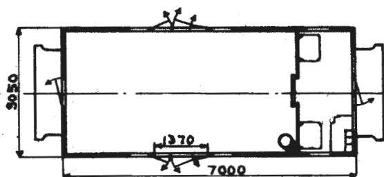
Grunnriss 1 Hovedt. 657
