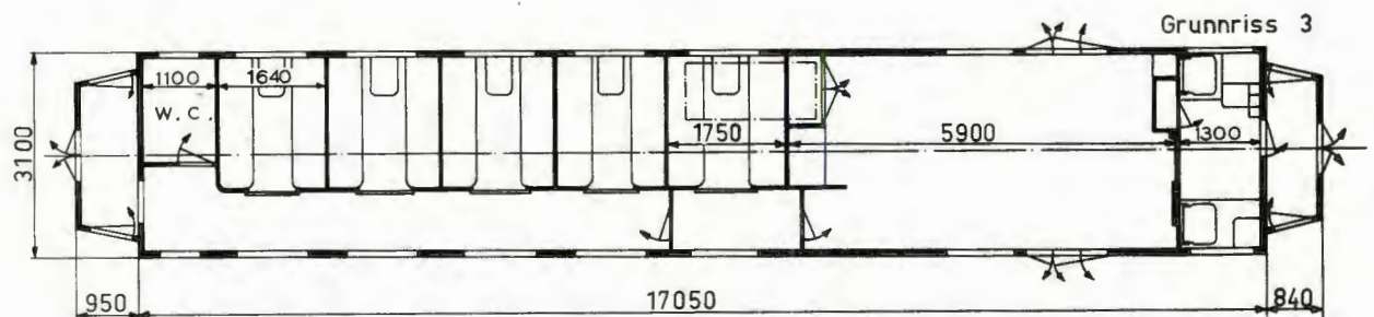
Hovedt. 1841
