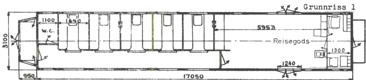
Hovedt. 2126
