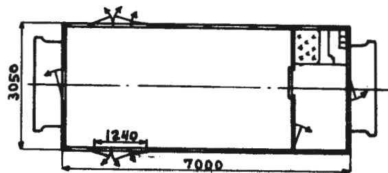
Grunnriss 2 Oppr. hovedt. 478
