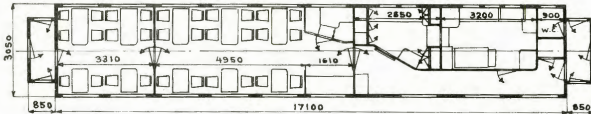
Hovedt. 925
