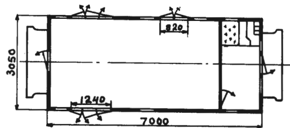
Grunnriss 1 Oppr. hovedt. 478
