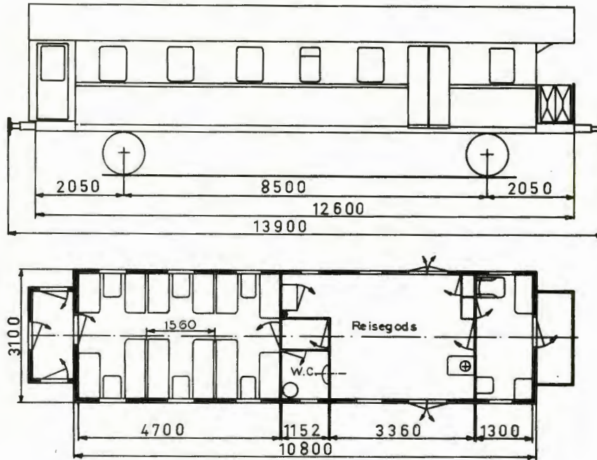
Hovedt. 7273
