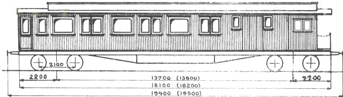
Mål i ( ) gjelder vogner etter grunnriss 2. og 3
