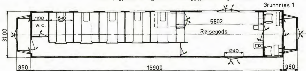
Hovedt. 3039
