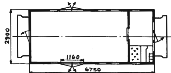
Grunnriss 2 Hovedt. 261
