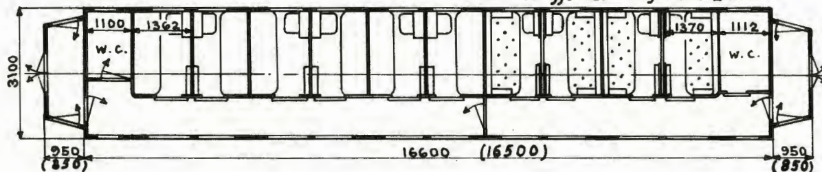
Mål i ( ) gjelder vogn nr. 207
