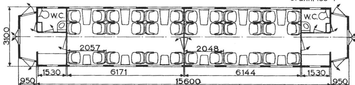
Oppr. hovedt. 2067 1)
