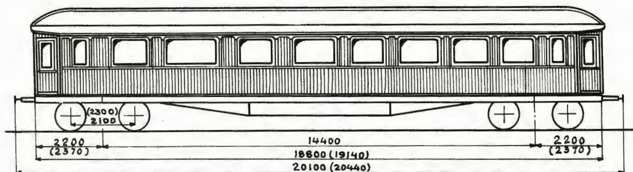
Måli ( ) gjelder vogner etter grunnriss 2.
