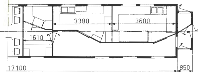
Hovedt. 2068 1)
