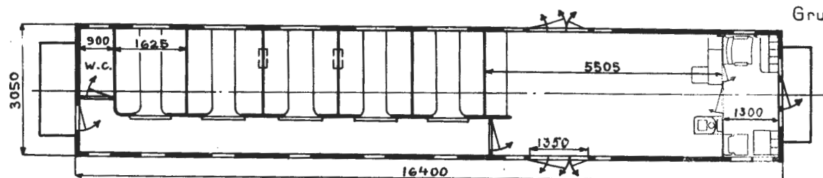
Hovedt. 502
