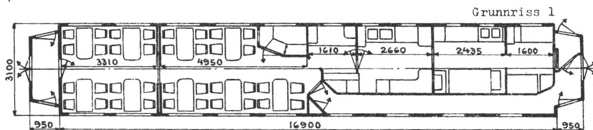
Hovedt. 2115
