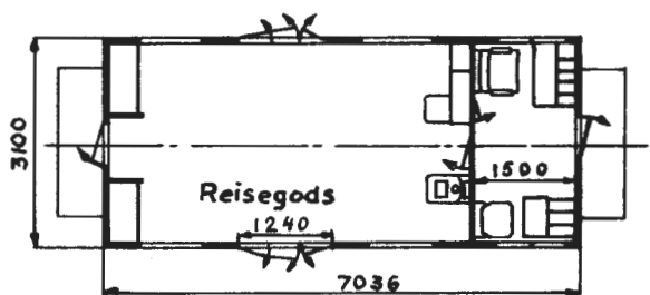
Grunnriss 2 Oppr. hovedt. 478 1) 992 1)
