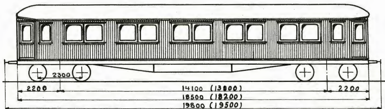
Mål i ( ) gjelder vogn nr. 207
