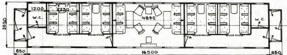
Hovedt. 1134
