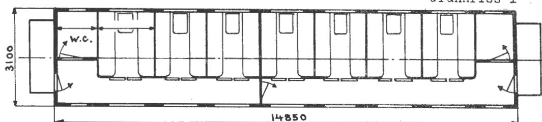
Oppr. hovedt. 312b
