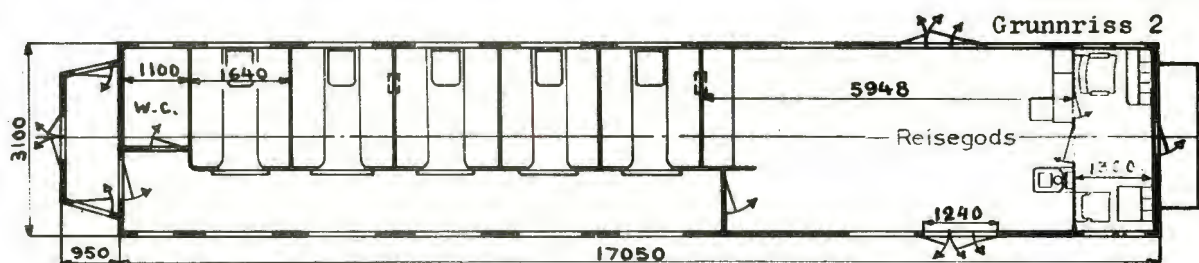
Hovedt. 2126
