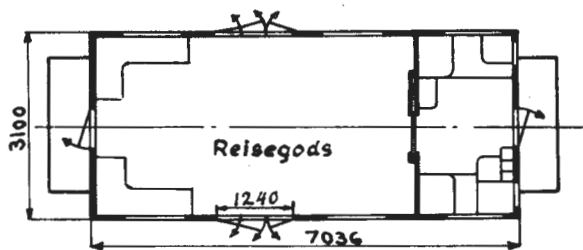
Grunnriss 1 Hovedt. B. 543
