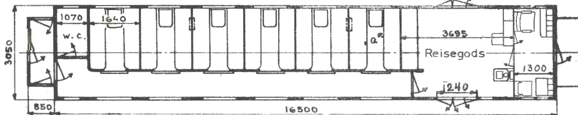
Hovedt. 1073
