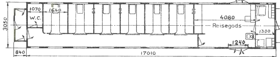
Hovedt. 1074
