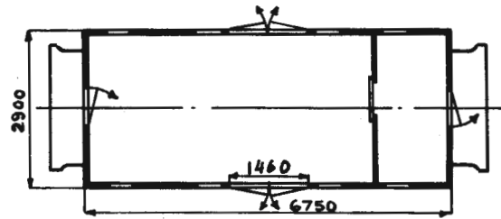
Grunnriss 1 Oppr. hovedt. 81
