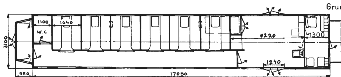
Hovedt. 3109
