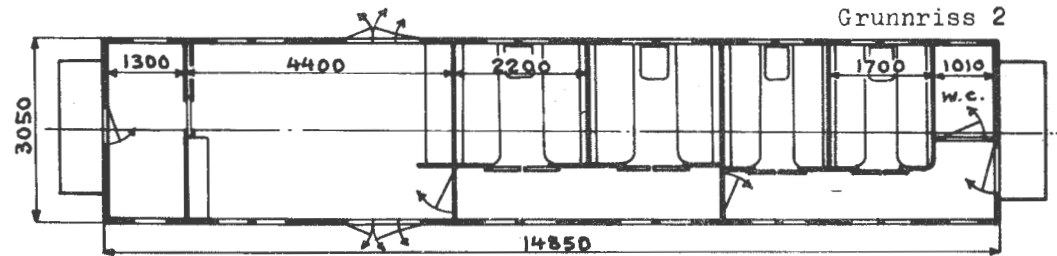
Oppr. hovedt. 7 1)
