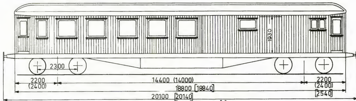
Mål i ( ) gjelder for grunnriss. Mål i [ ] gjelder for grunnriss 3
