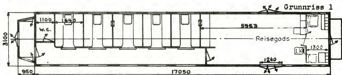
Hovedt. 2126
