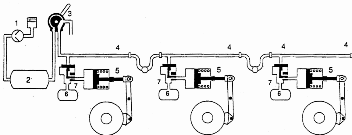
Bremsestilling
