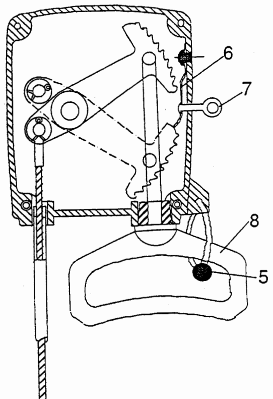
Nødbremsehåndtak
