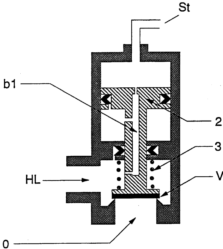
Pneumatisk nødbremseventil
