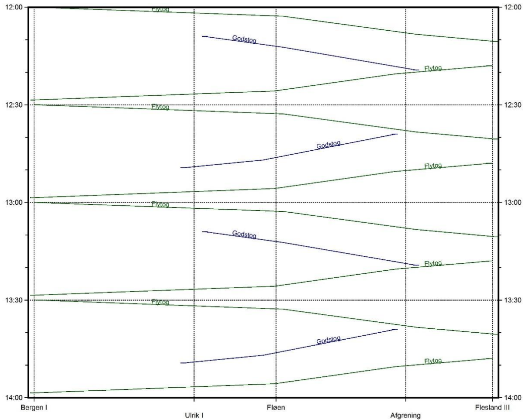
Figur 3-3 Eksempel på grafisk ruteplan Bergen - Fløyen - Flesland, med Flytog i halvtimesdrift og godstog i mellom Ulrikstunnelen og sporvekslingen mot Logistikk-knutepunktet i tidedrift.
