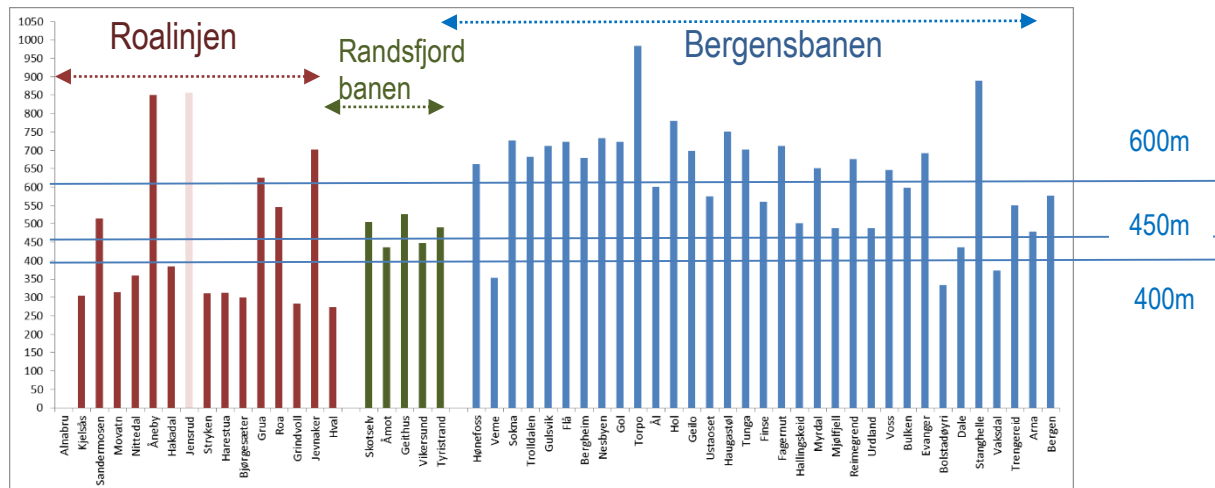
Figur 3-27. Oversikt over lengde på dagens kryssingsspor på Roalinjen, Randsfjordbanen og Bergensbanen. Kilde: Jernbaneverket
