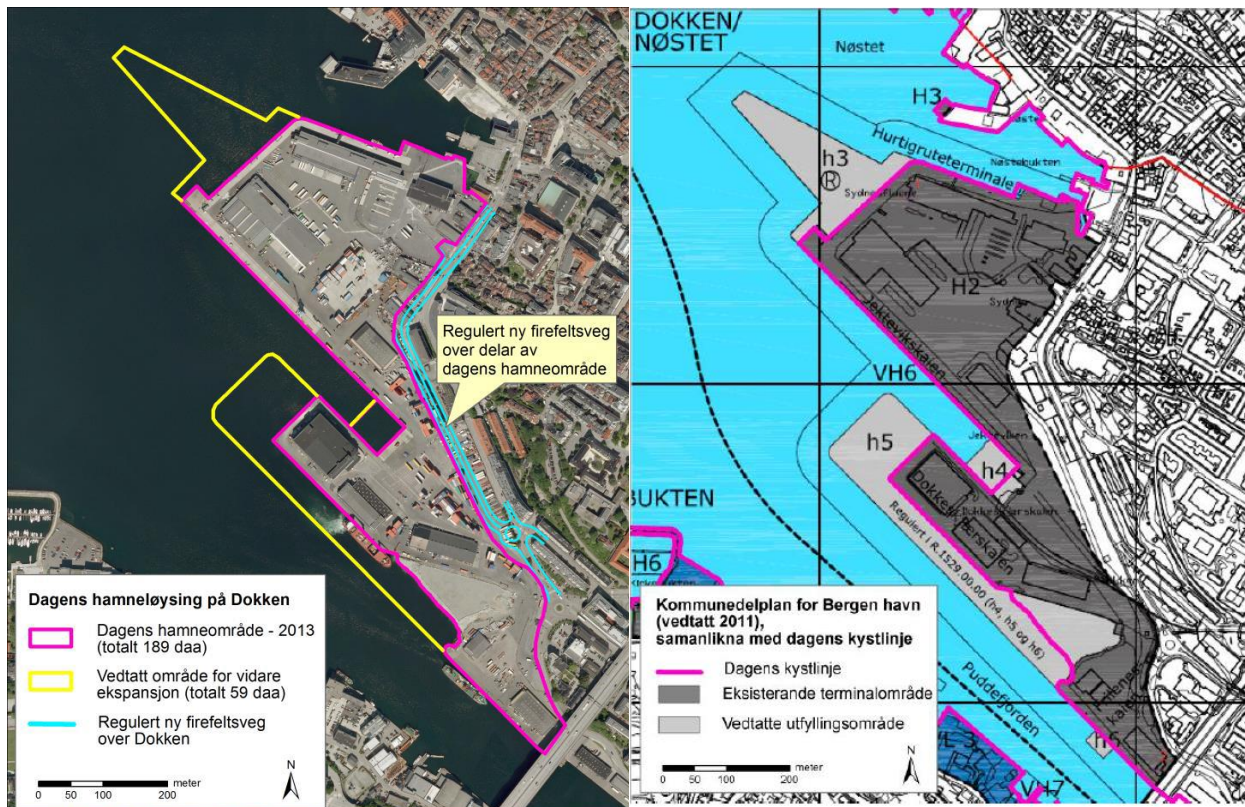
Figur 3-38. Illustrasjon av dagens havneløsning på Dokken. Kilde: Vedlegg til planprogram for ny godshavn i Bergensområdet, 10.okt.2013.
