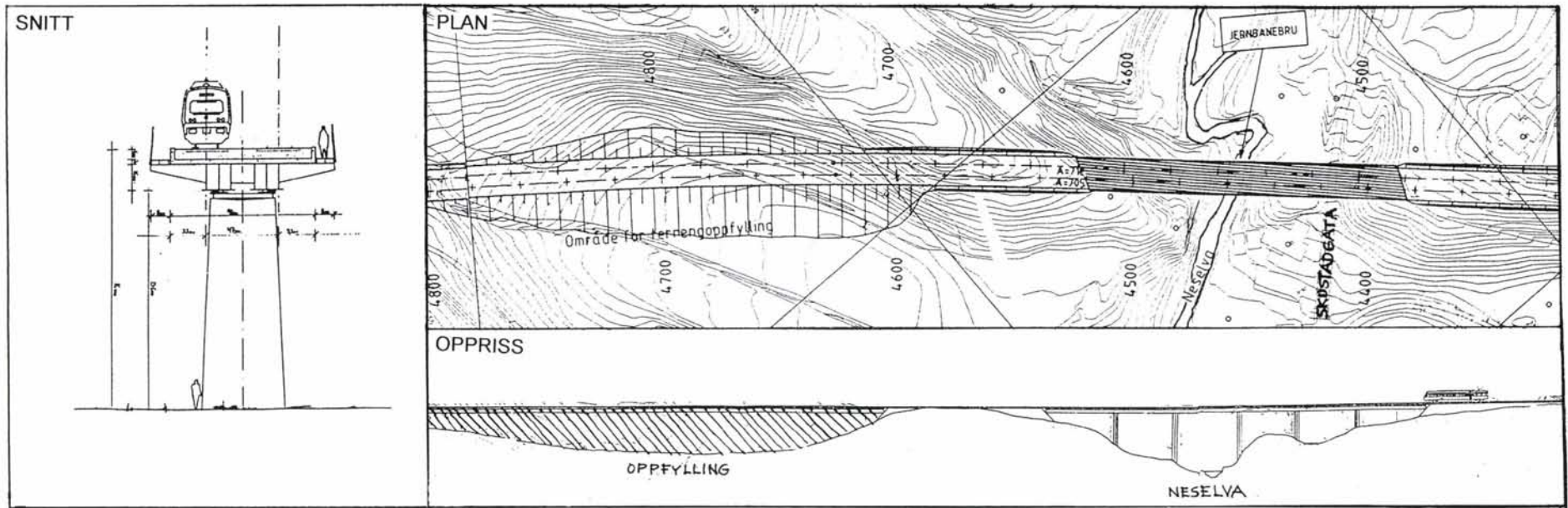
Fig. 8.10.2 Snitt, plan og oppriss for jernbanebru over Neselva. Alternativ Ytre linje.
