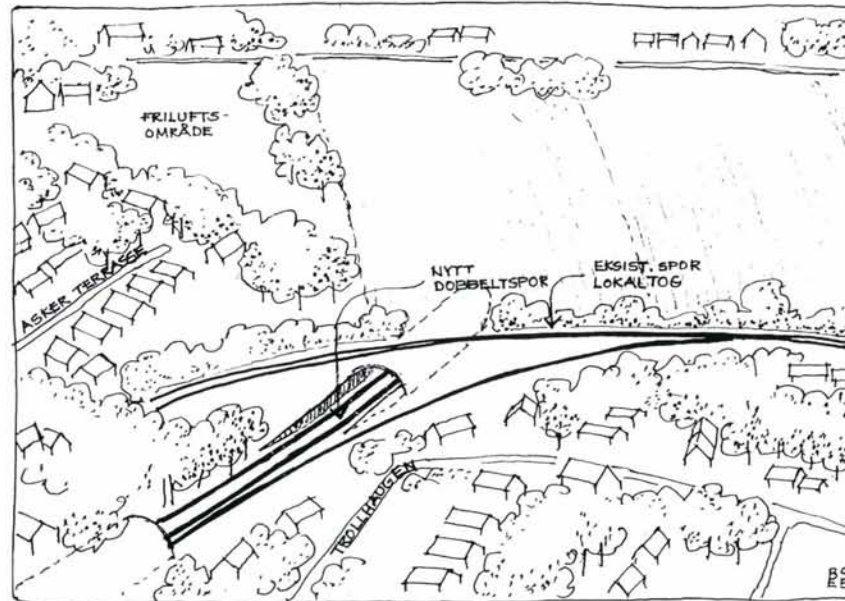
Fig. 8.11.2 Det nye dobbeltsporet vil gå dels i kulvert og dels i nedsenket, åpen sone.
