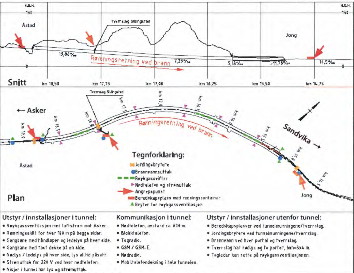
Figur 7: Tanumtunnelen - særskilt brannobjekt, beredskapstegning.
