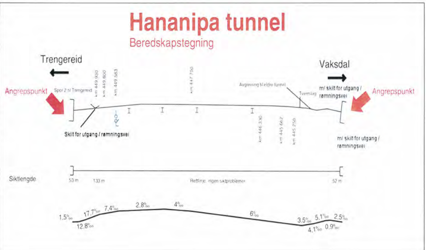
Figur 21: Hananipa tunnel - særskilt brannobjekt, beredskapstegning.
