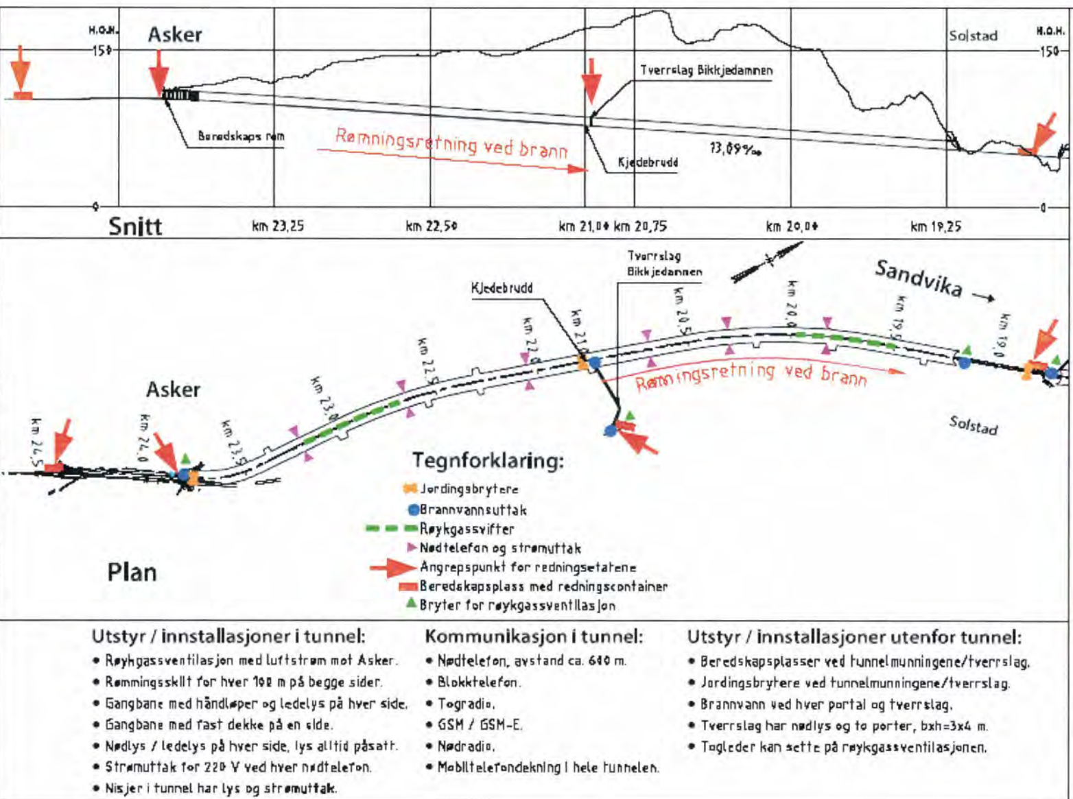
Figur 8: Skauguntunnelen - særskilt brannobjekt, beredskapstegning.
